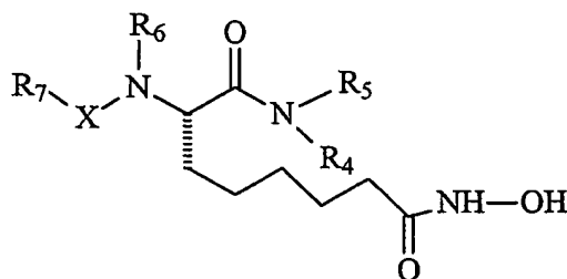
(IIIb)
